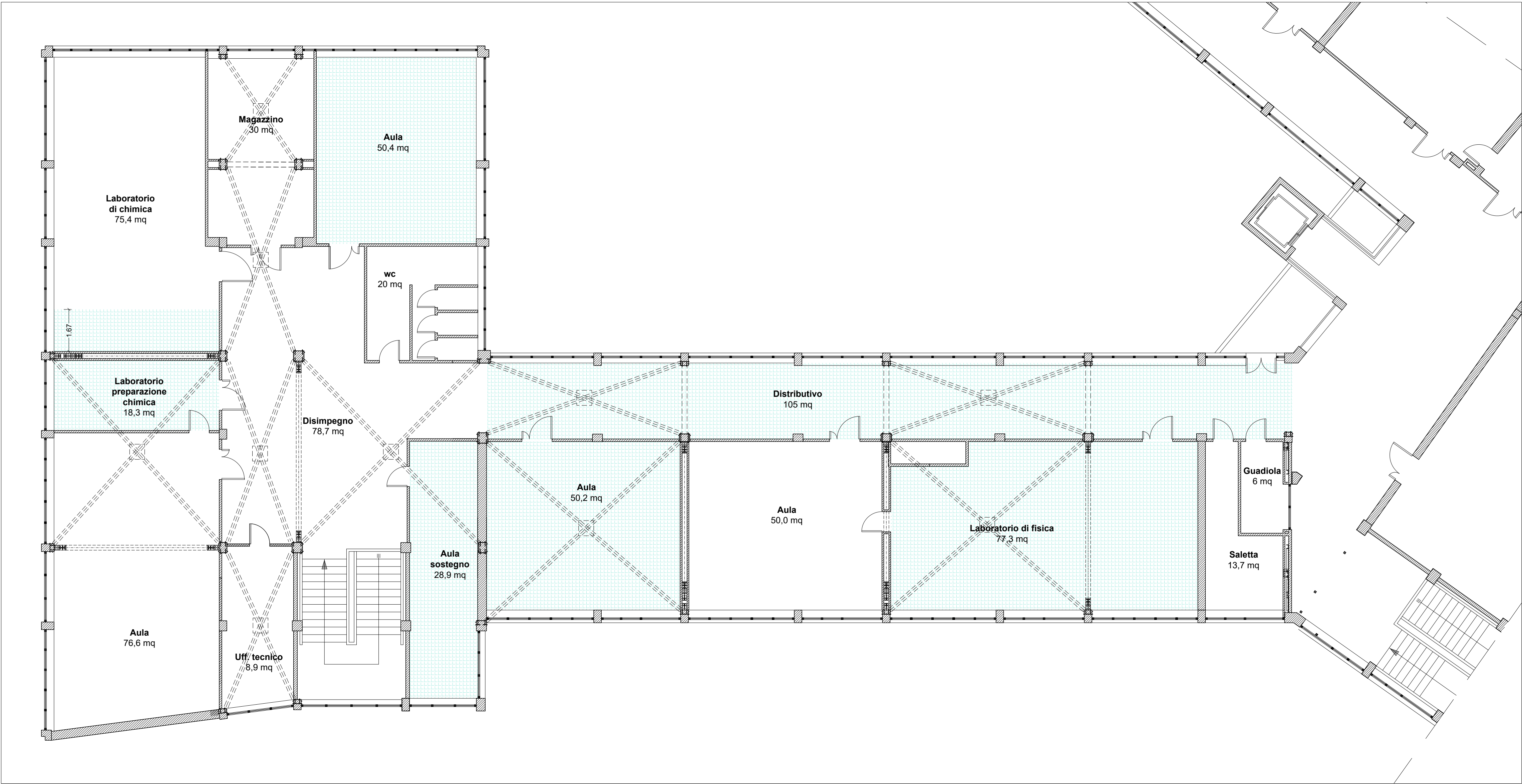
Pianta dei controsoffitti - piano secondo scala 1:100
